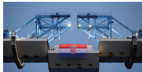
图 3：佩列沙茨跨海大桥的最后一块钢箱梁被缓缓吊起
